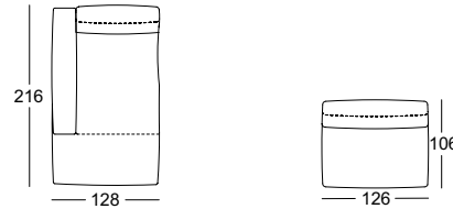
Übertiefe-Abschluss-Anreihbank*
